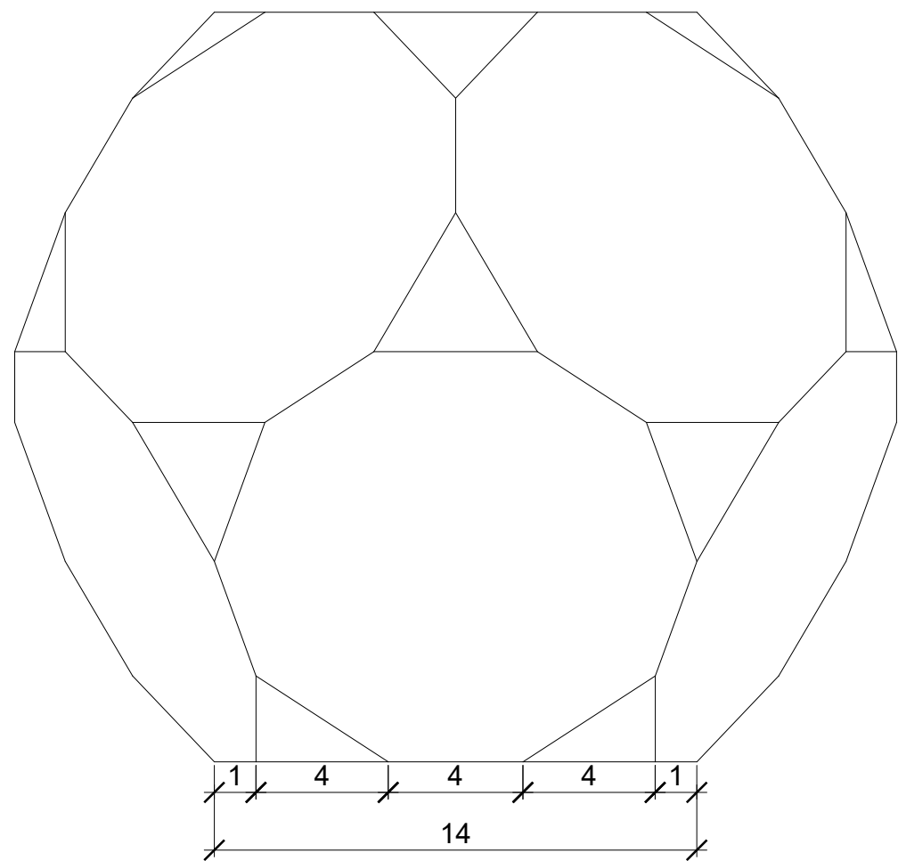
Alçado Frontal Esc. 1/2
