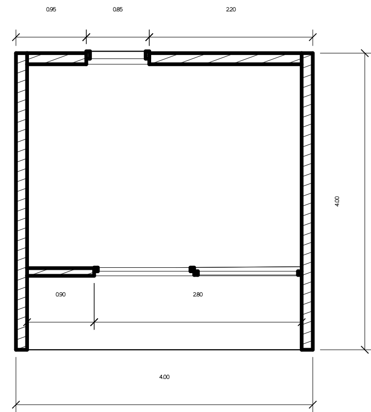
PLANTA TÉRREA
