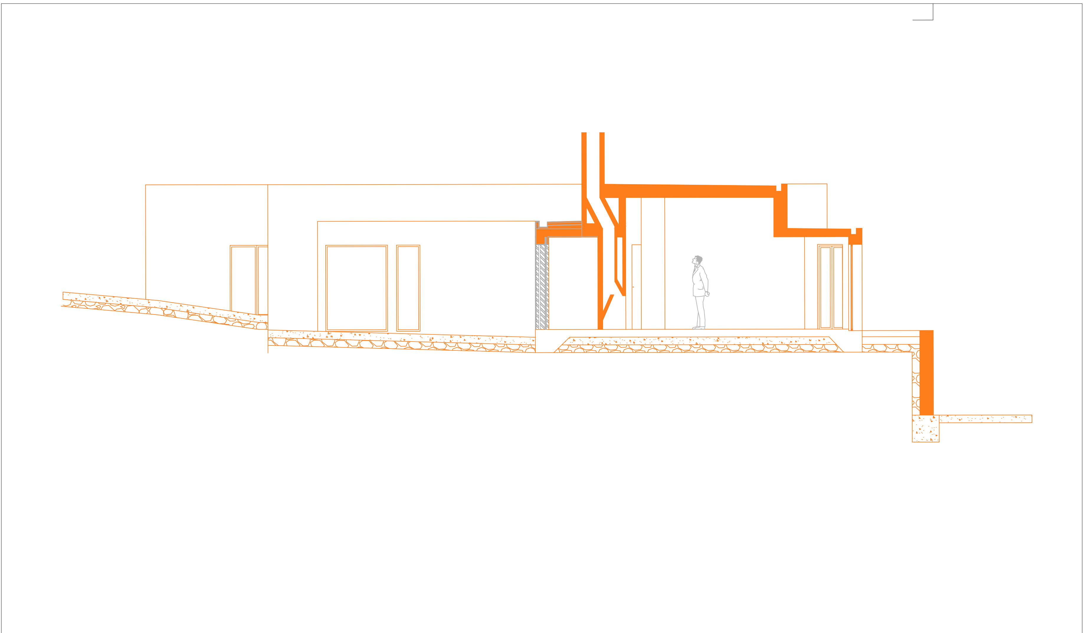
Corte A
