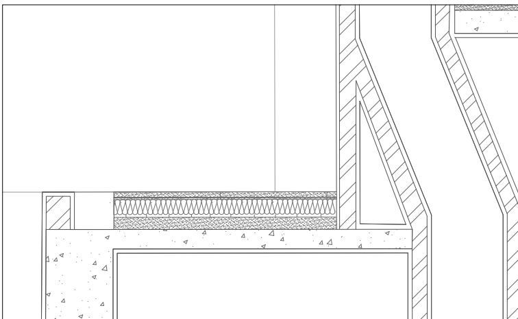
Pormenor cobertura 1:5
