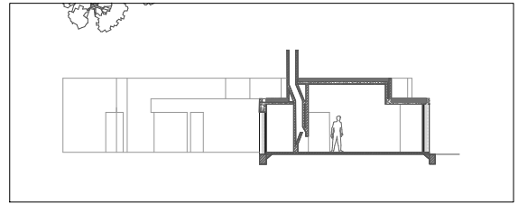
Corte 1:100
