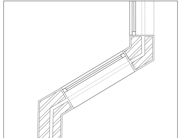
Pormenor janela 1:5
