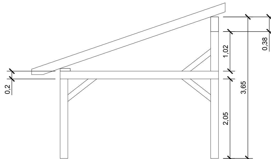
Alçado Lateral
