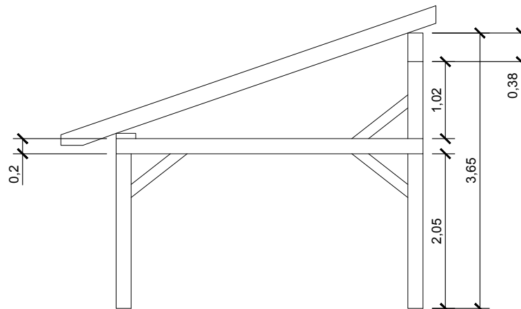
Alçado Lateral
