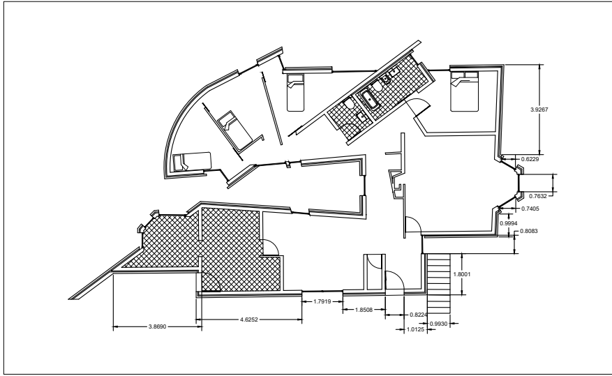
Planta 1:100
