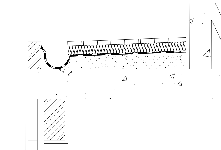
Pormenor Cobertura 1:10
