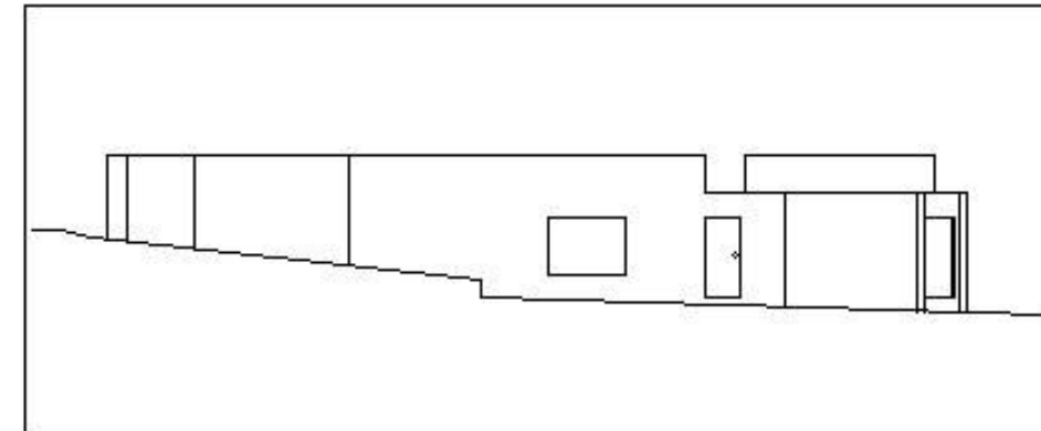
Alçado Sudoeste 1:100
