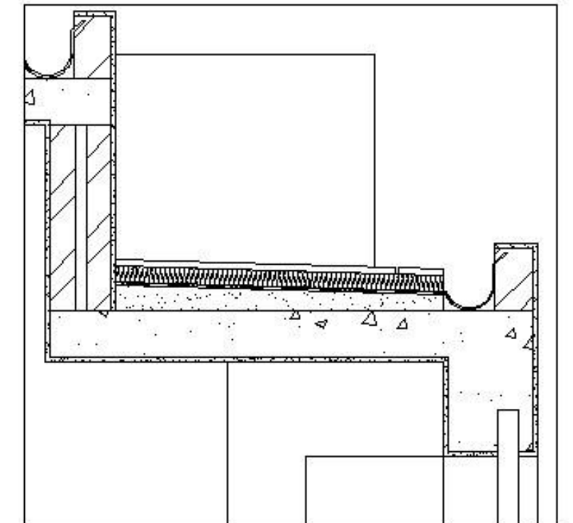
Promenor cobertura 1:5
