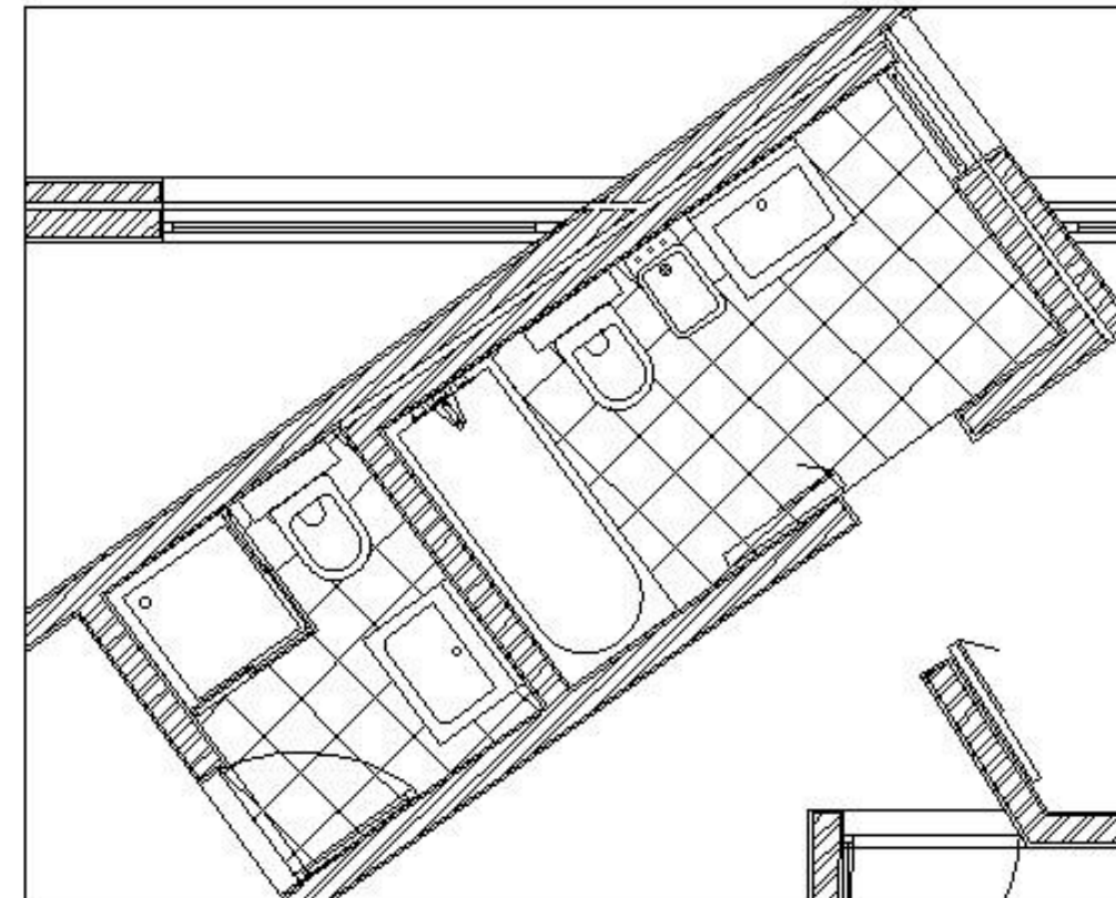
Promenor casa de banho 1:20
