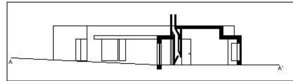
Corte longitudinal AA' 1:100
