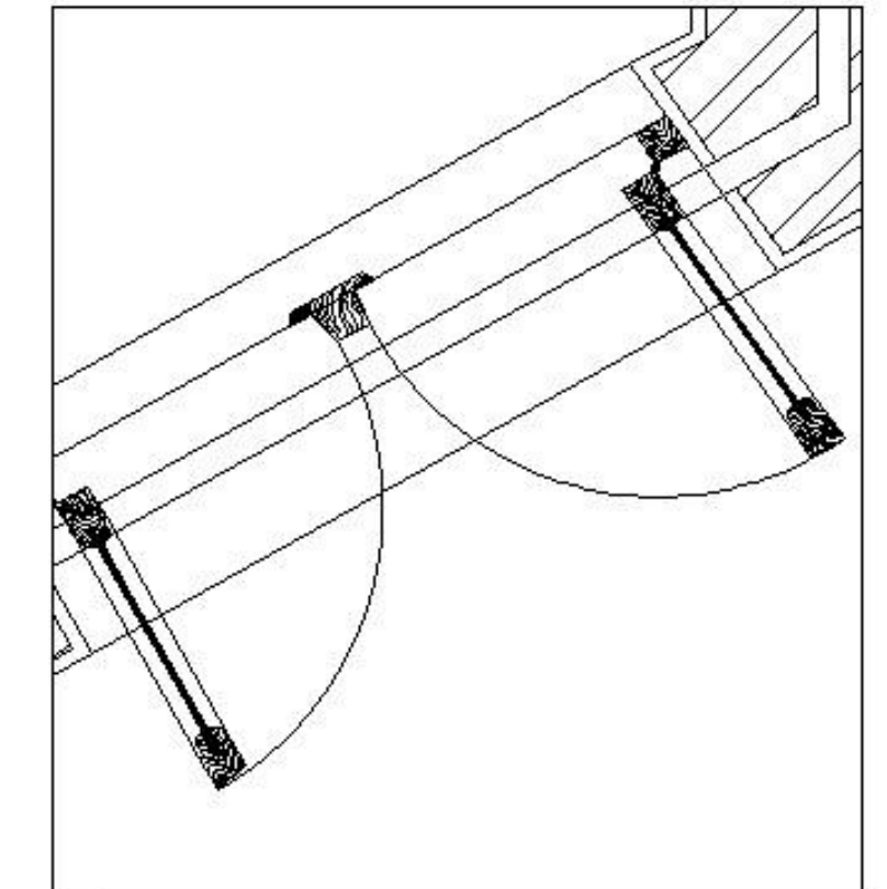
Detalhe caixilharia 1:5
