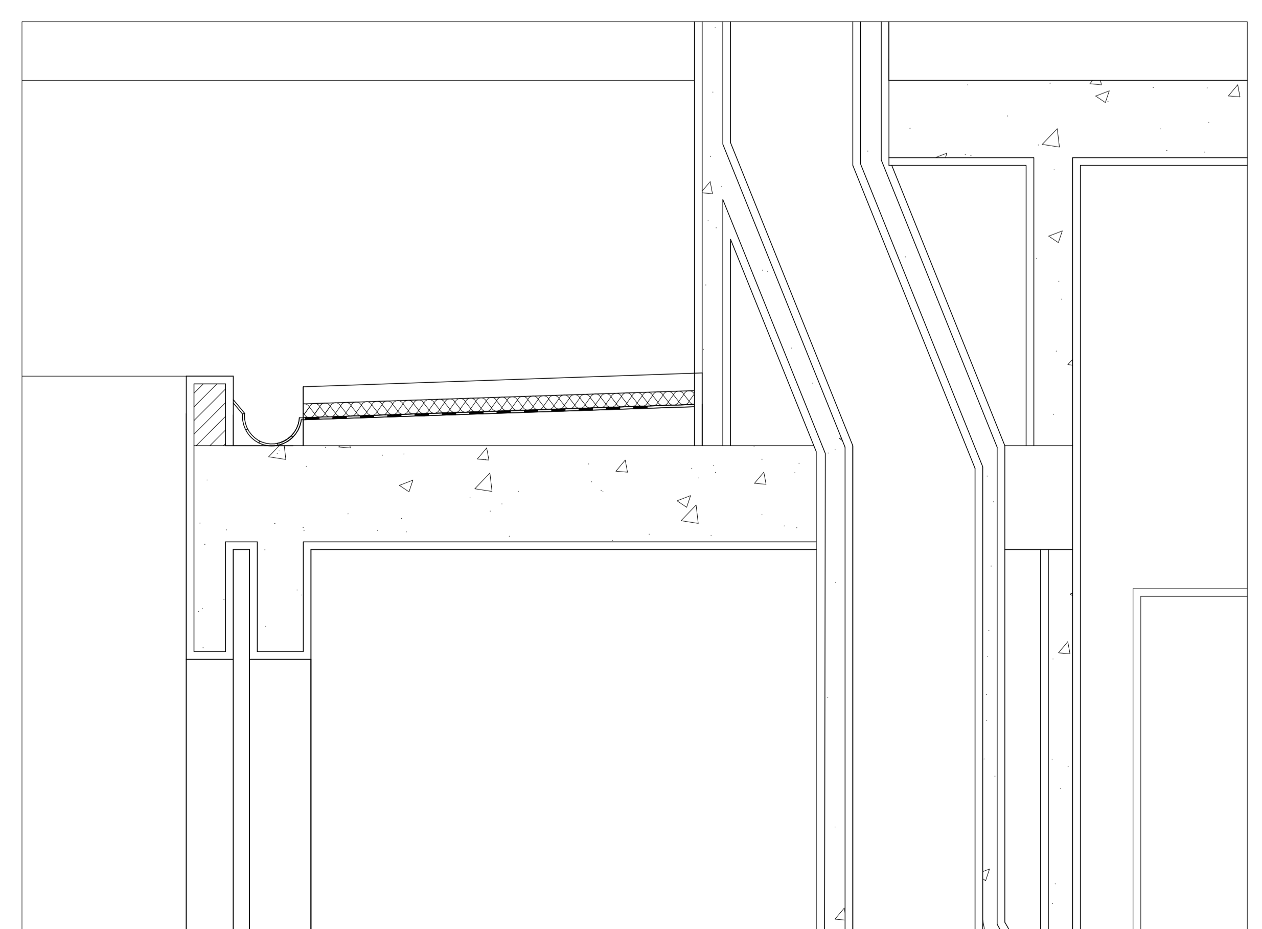
Extrato do Corte à escala 1/10
