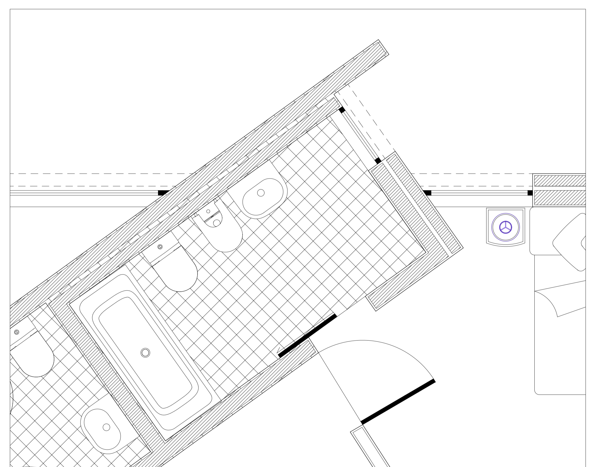
Extrato da Planta à escala 1/20
