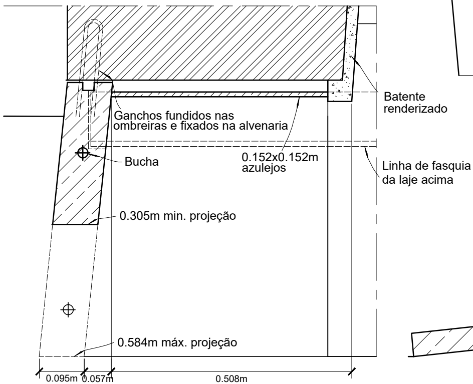
Secção vertical de fixação da moldura
