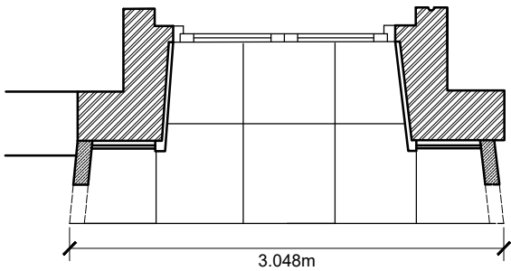
Planta escala 1/48
