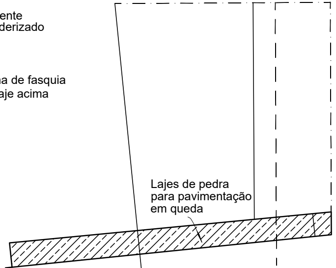
Secção vertical de fixação da moldura
