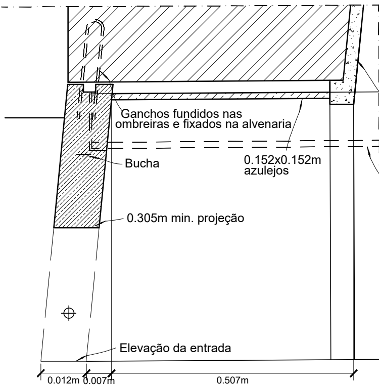
Plano de entrada escala 1/8
