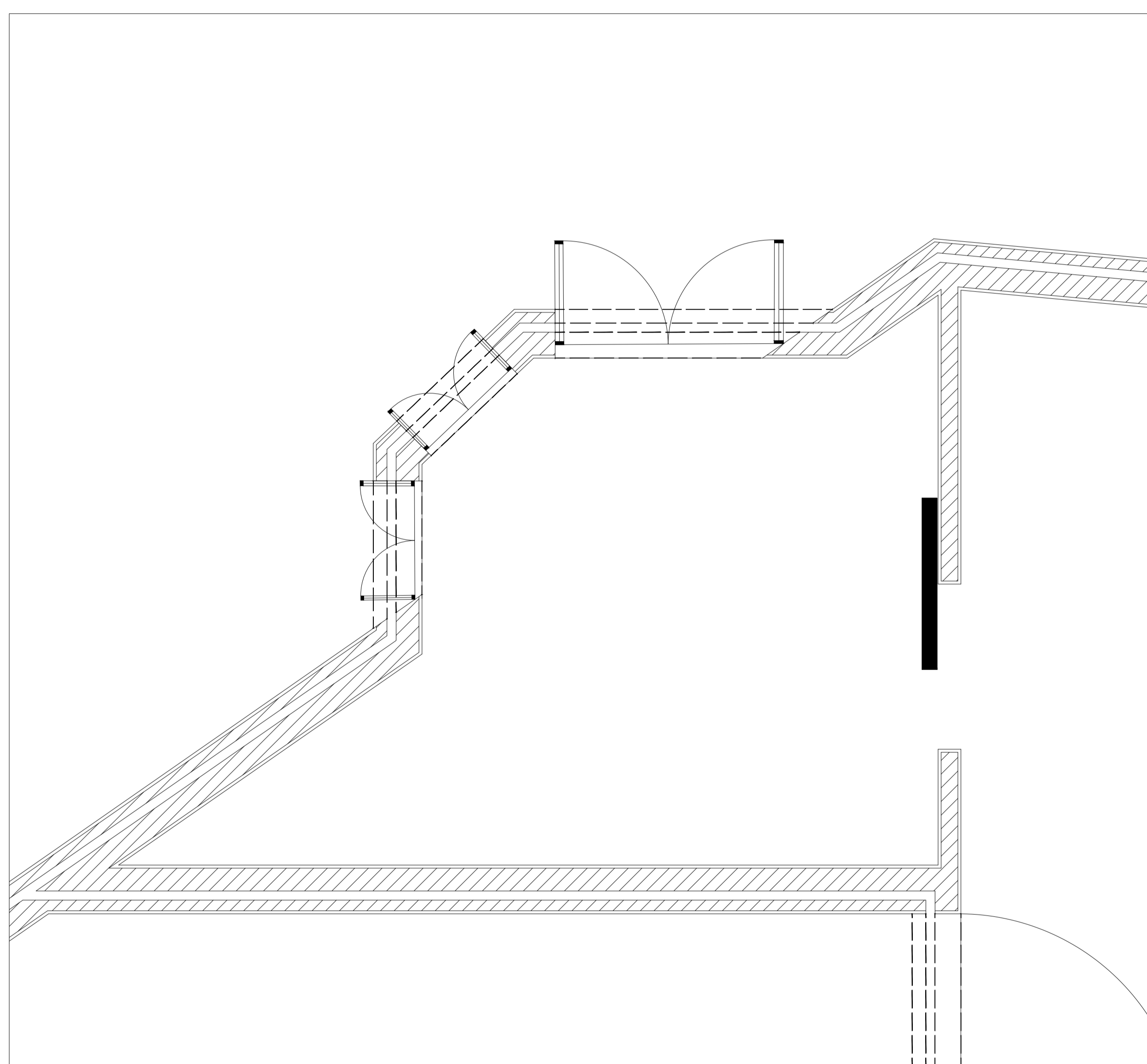
Detalhe (1/20)
