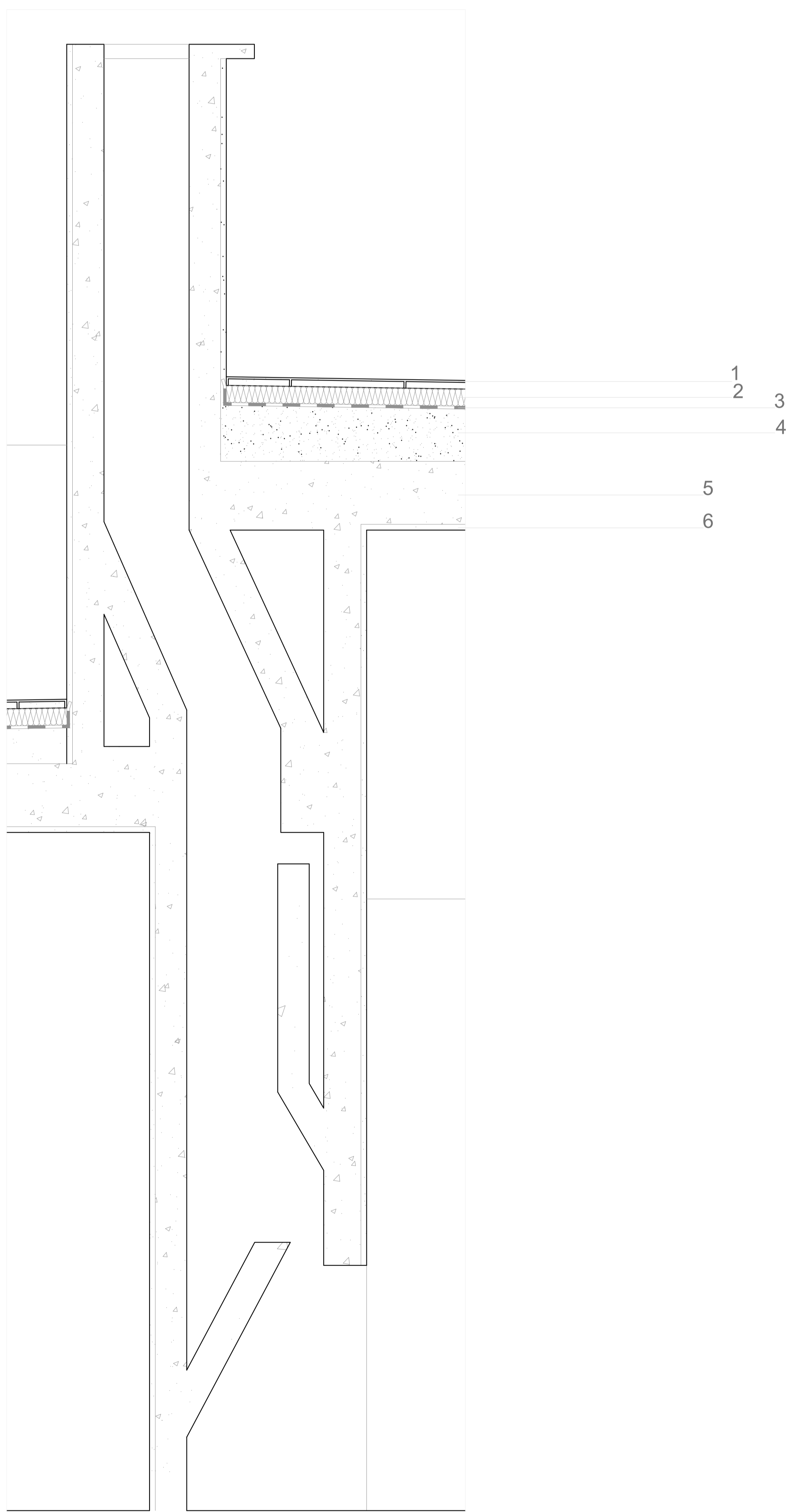
PORMENOR - CORTE CHAMINÉ ESCALA 1:10
