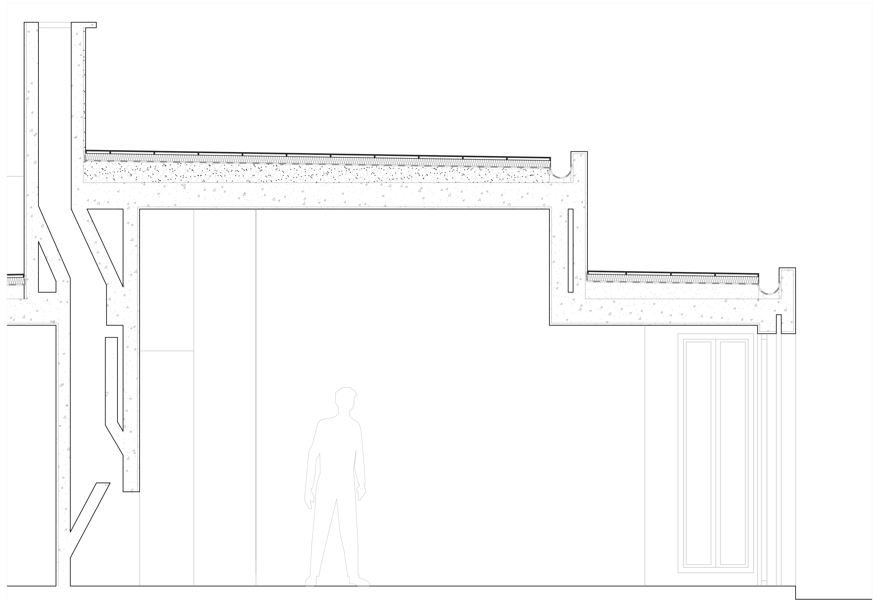
PORMENOR - CORTE ESCALA 1:20
