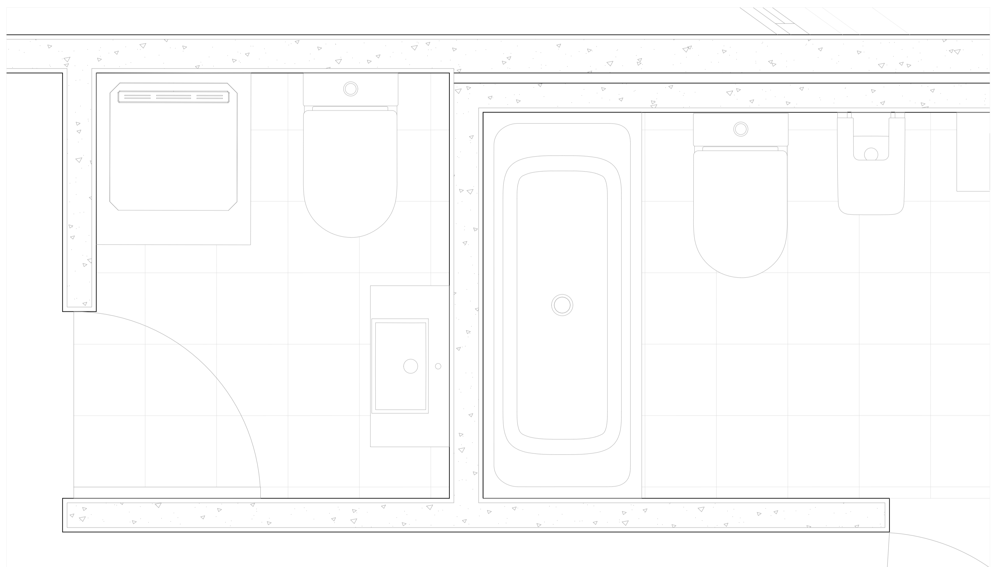
PORMENOR - CASA DE BANHO ESCALA 1:10
