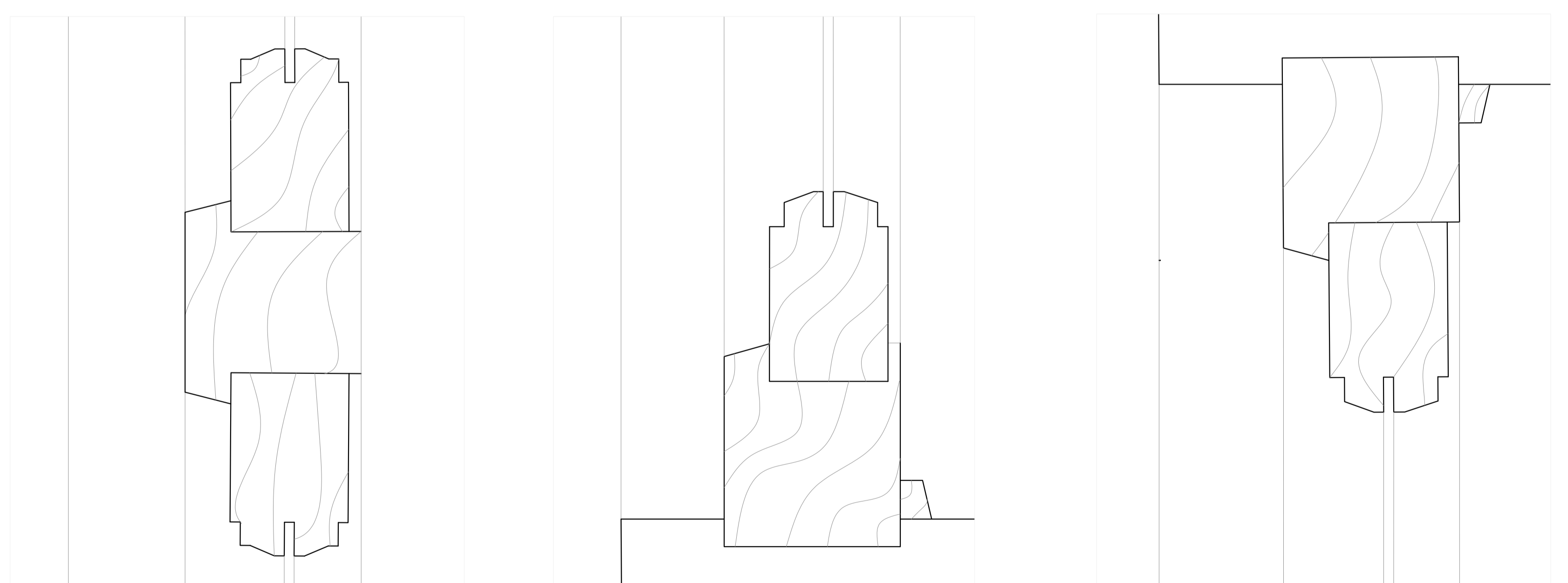
PORMENOR - CAIXILHARIA ESCALA 1:1
