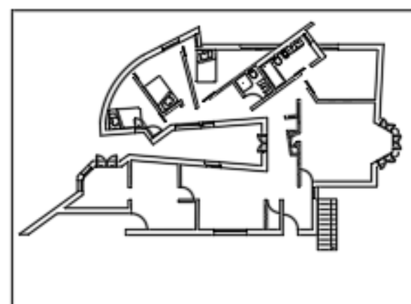
PLANTA 1:100
