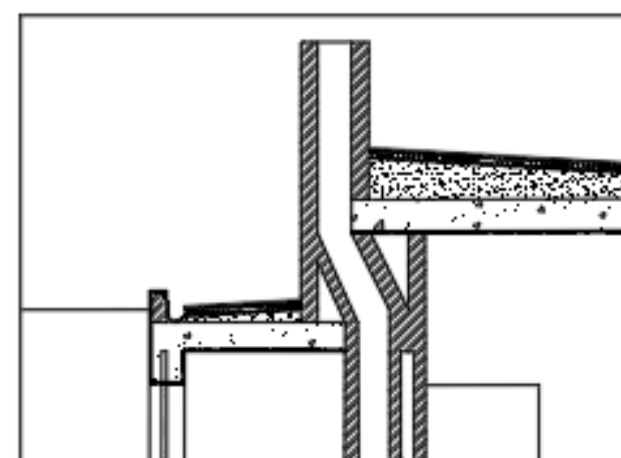
PORMENOR CORTE 1:20
