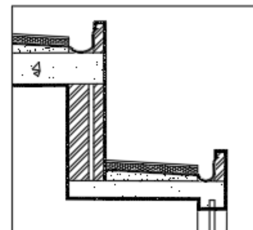
PORMENOR DE CORTE 1:10
