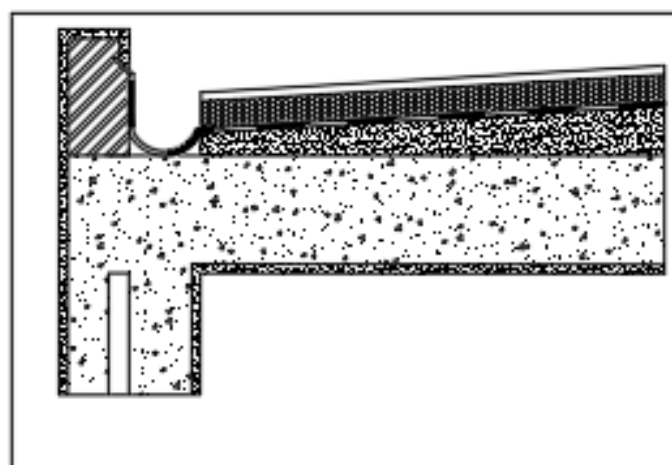
PORMENOR DE CORTE 1:5
