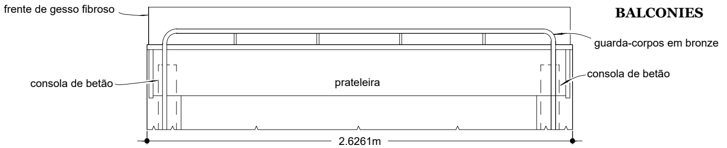
Planta da frente do camarote do auditório Escala: 1/24
