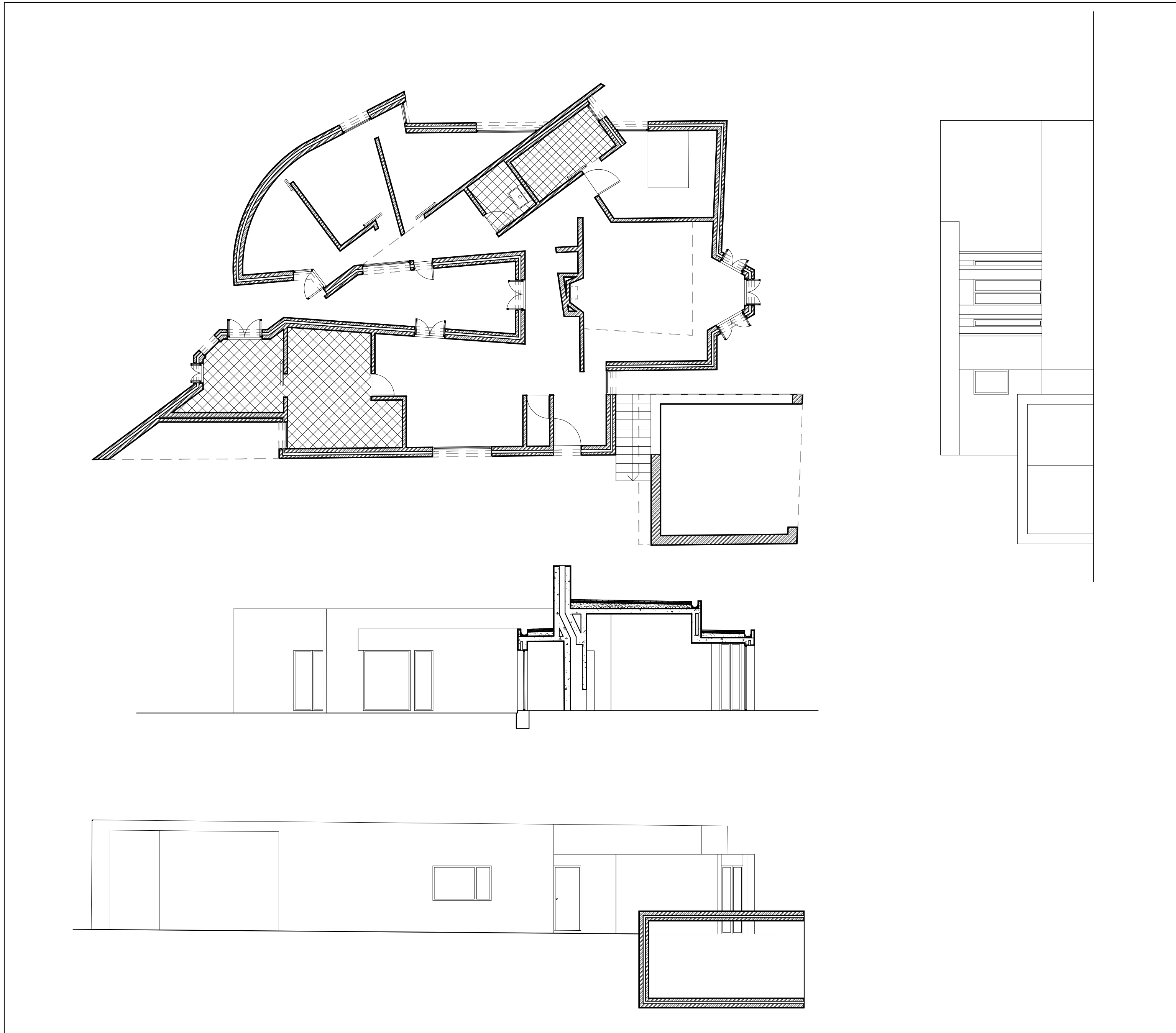
Planta, Corte e Alçados à escala 1:100
