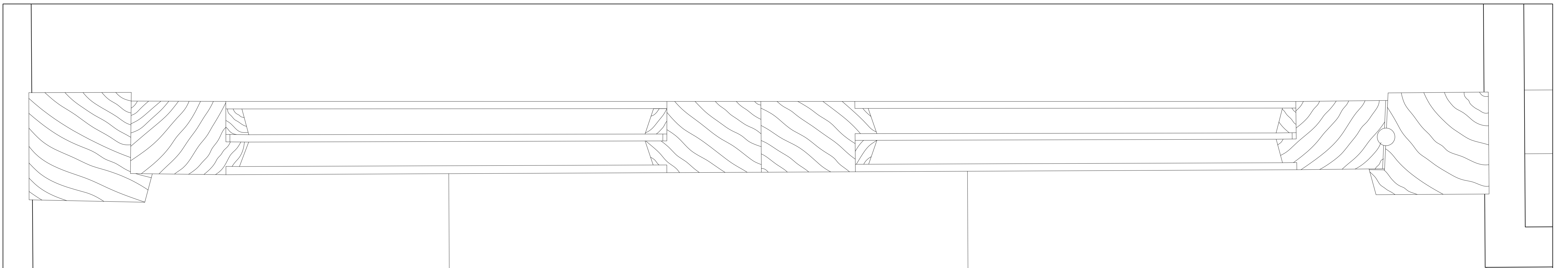
Detalhe Caixilharia de Madeira à escala 1:1
