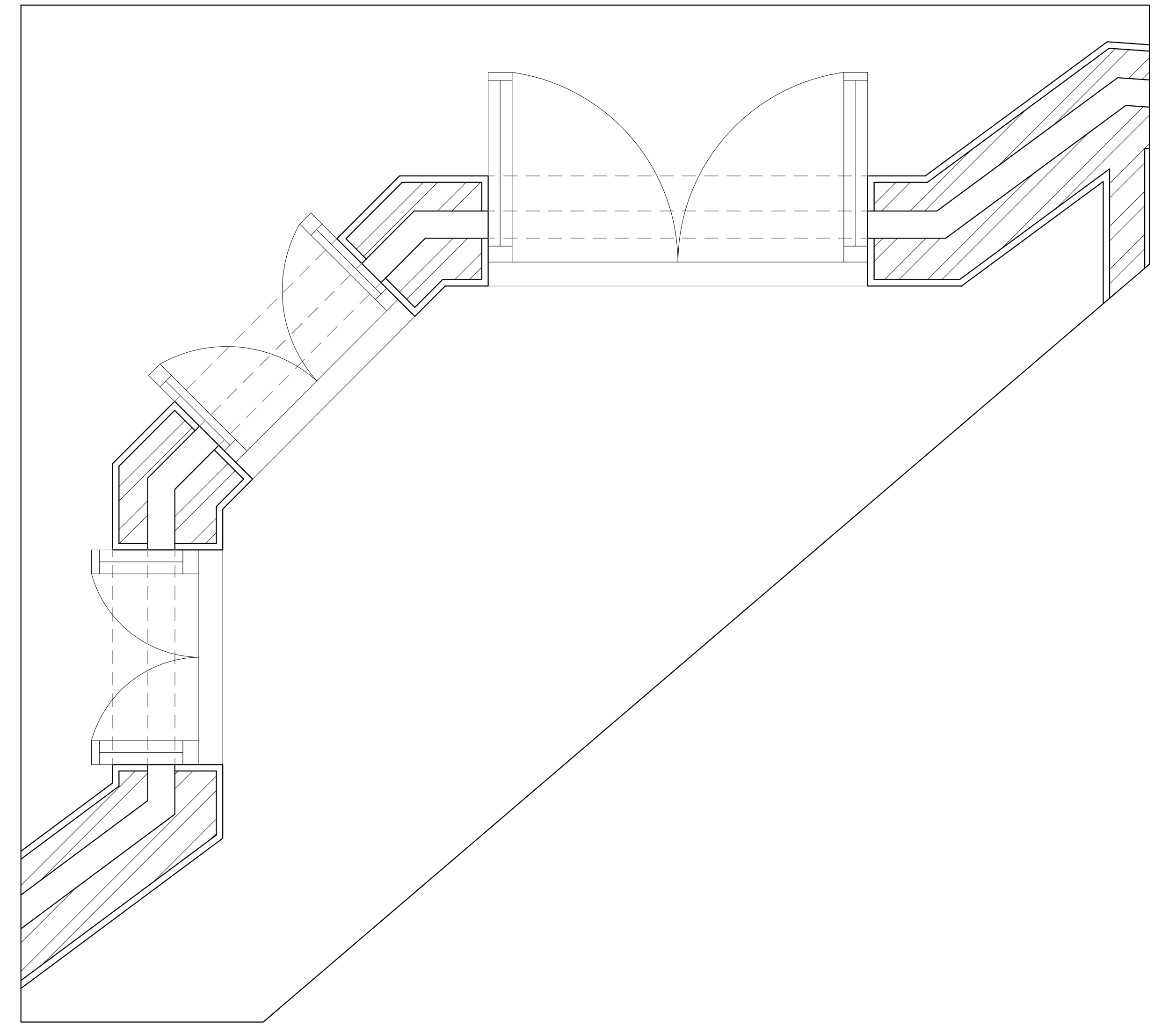
Detalhe Janela à escala 1:10
