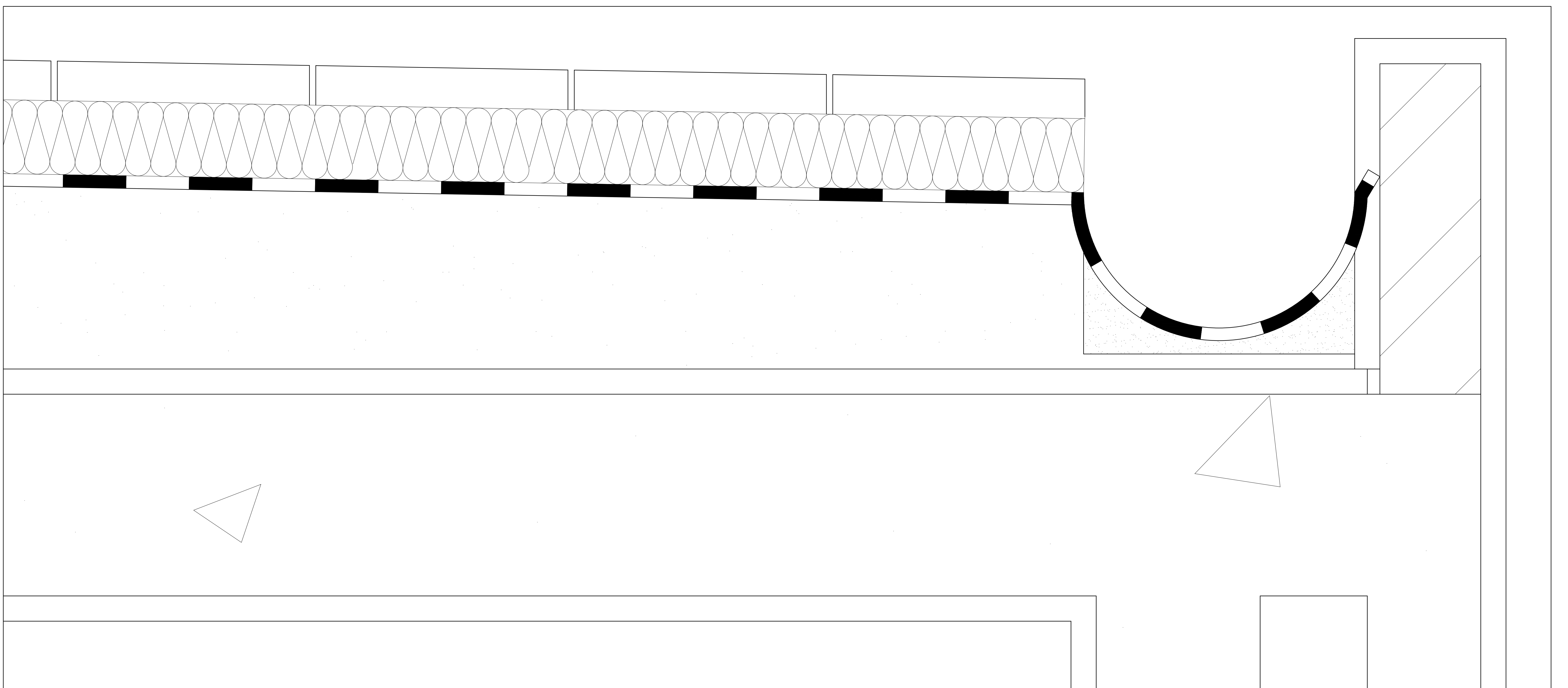
Detalho Telhado à escala 1:1
