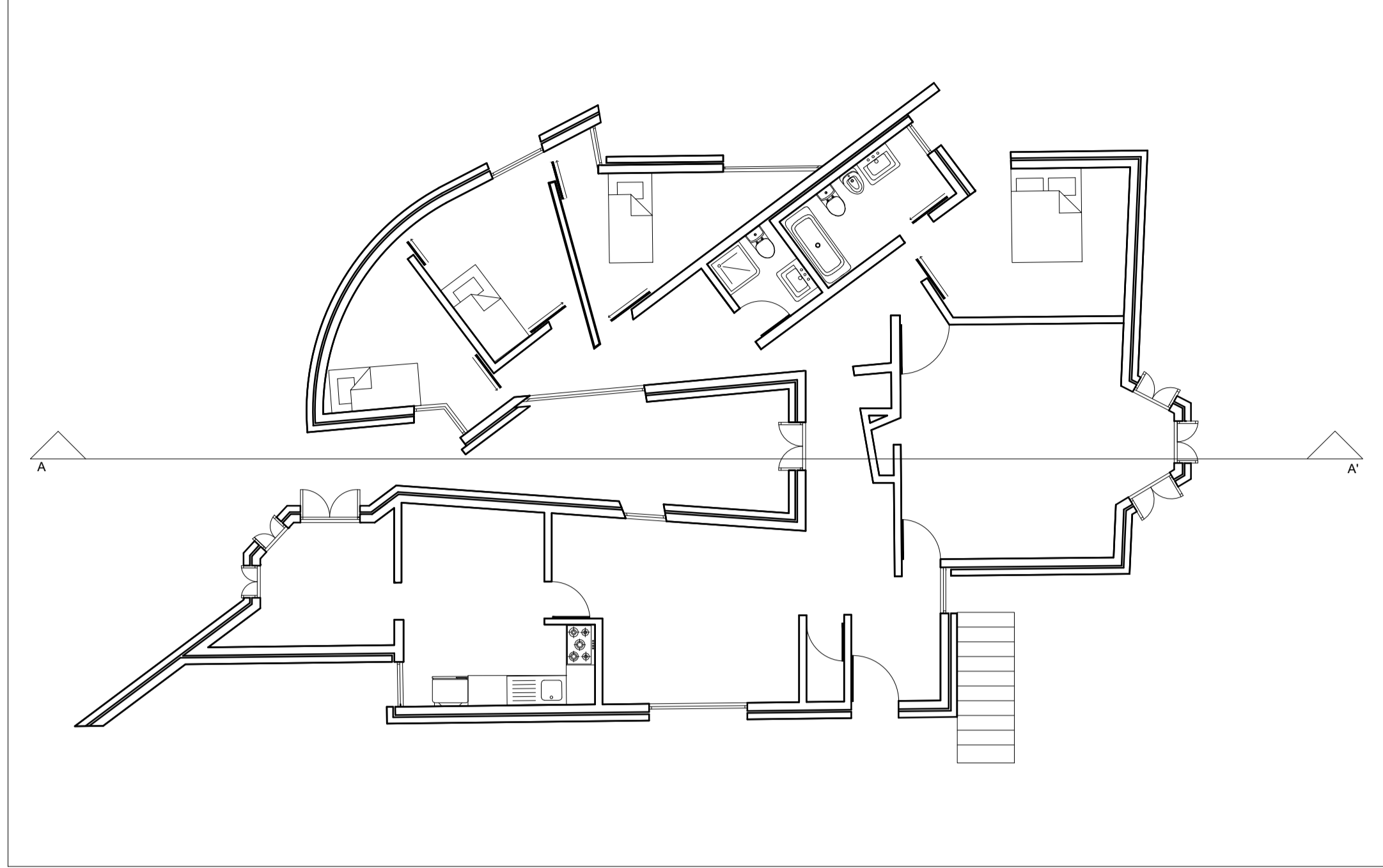
PLANTA 1:100
