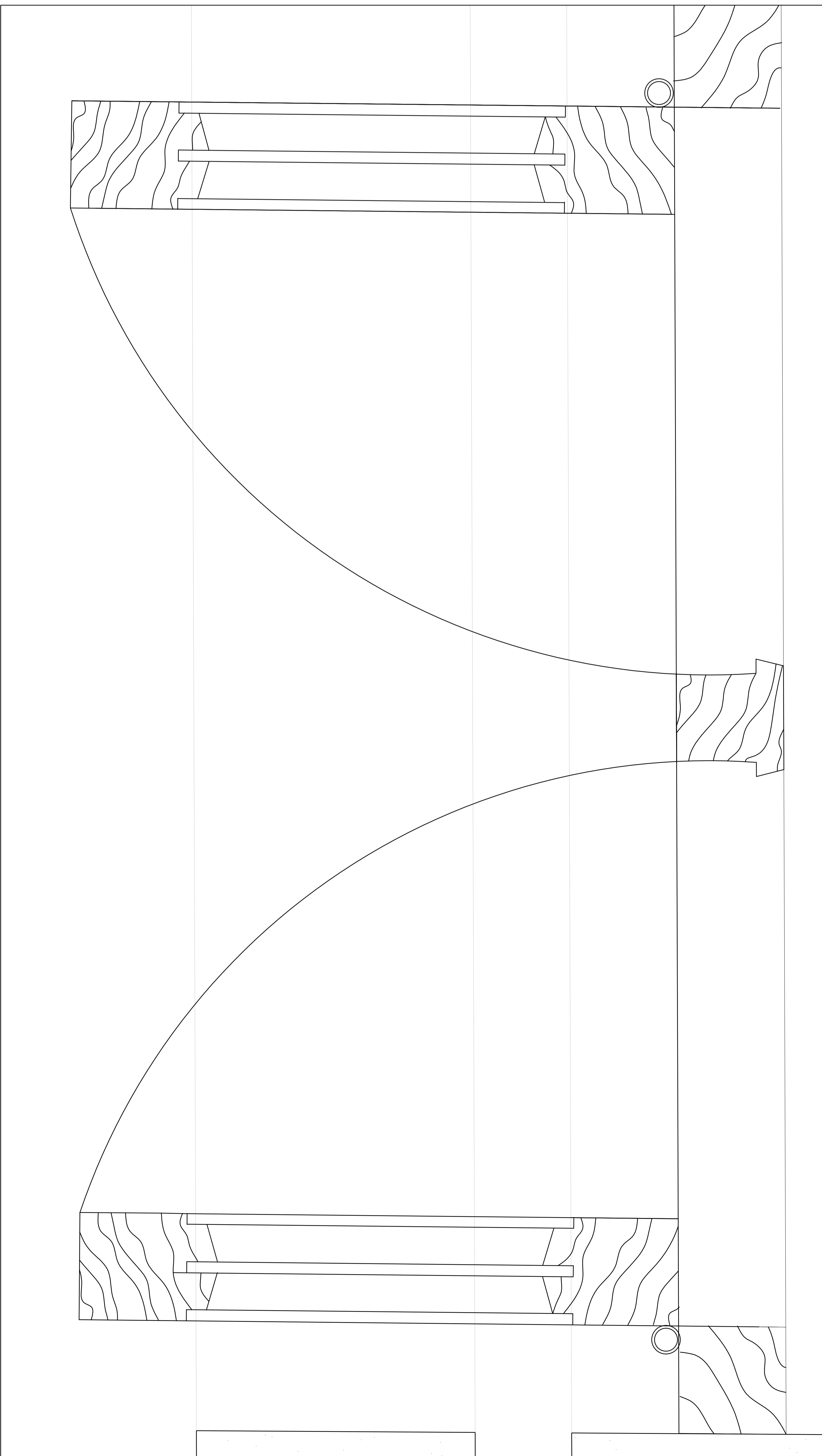
PORMENOR 1:1
