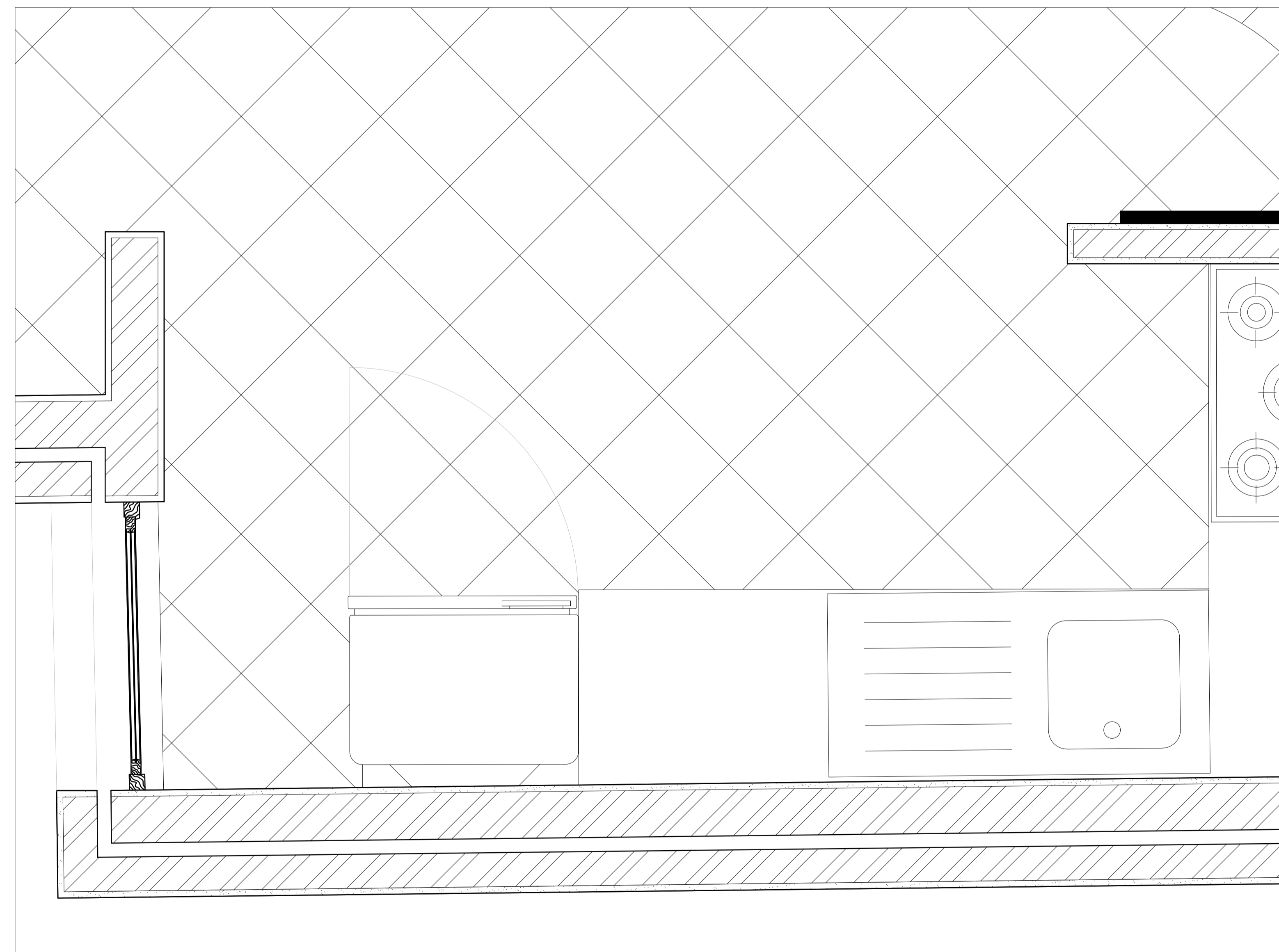
PORMENOR DA COZINHA 1:10
