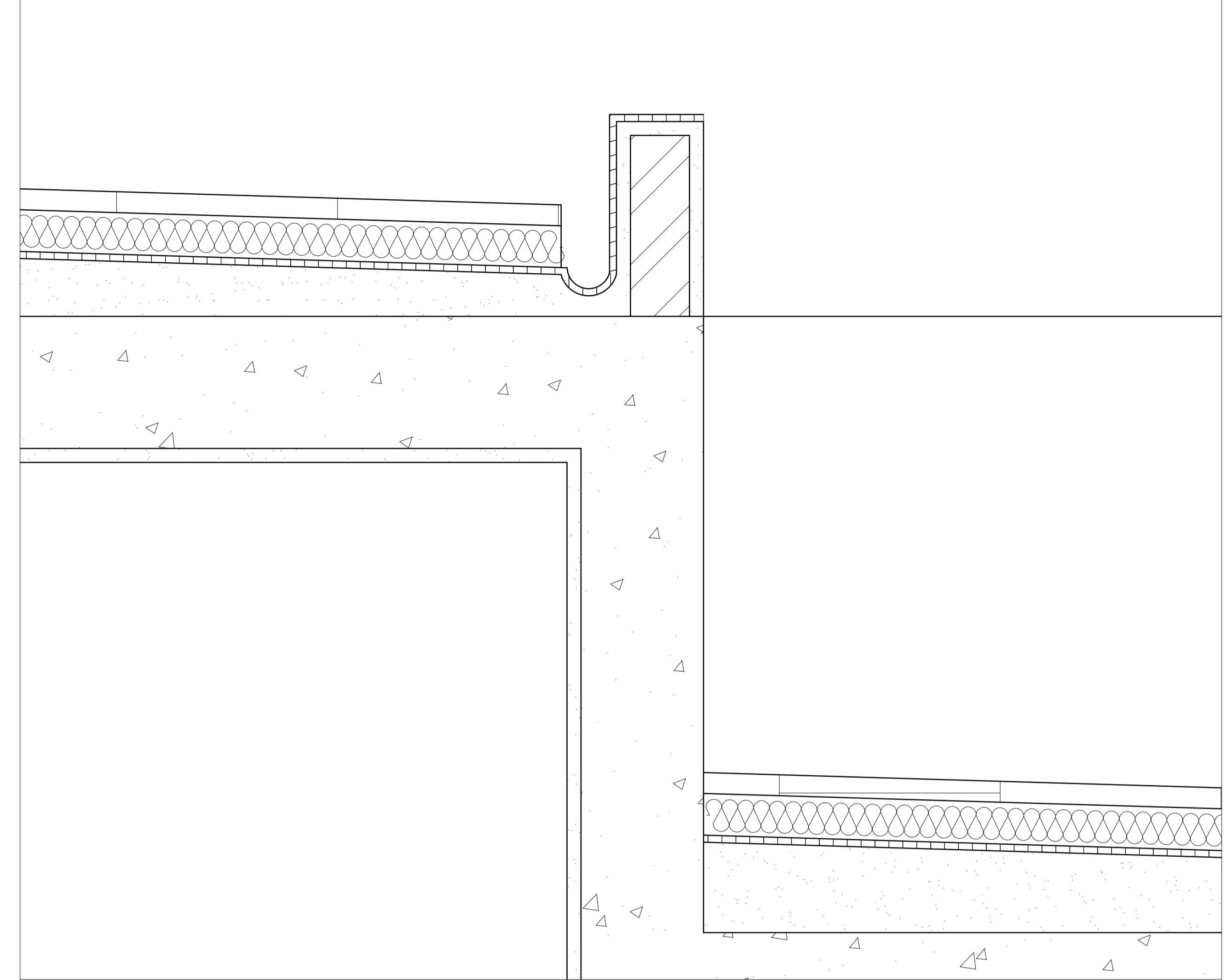
PORMENOR DA COBERTURA 1:5
