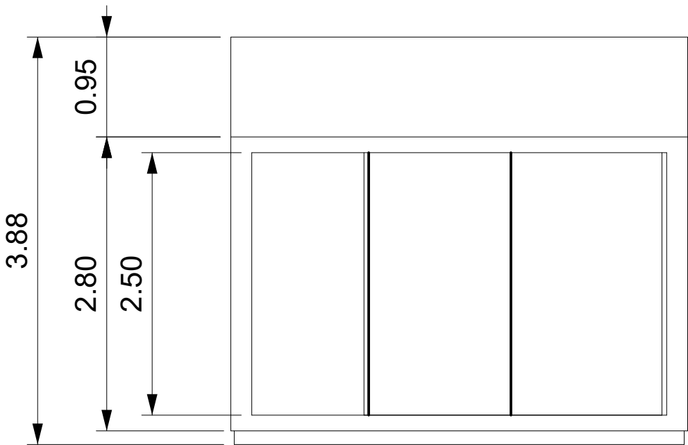
Alçado Sul
