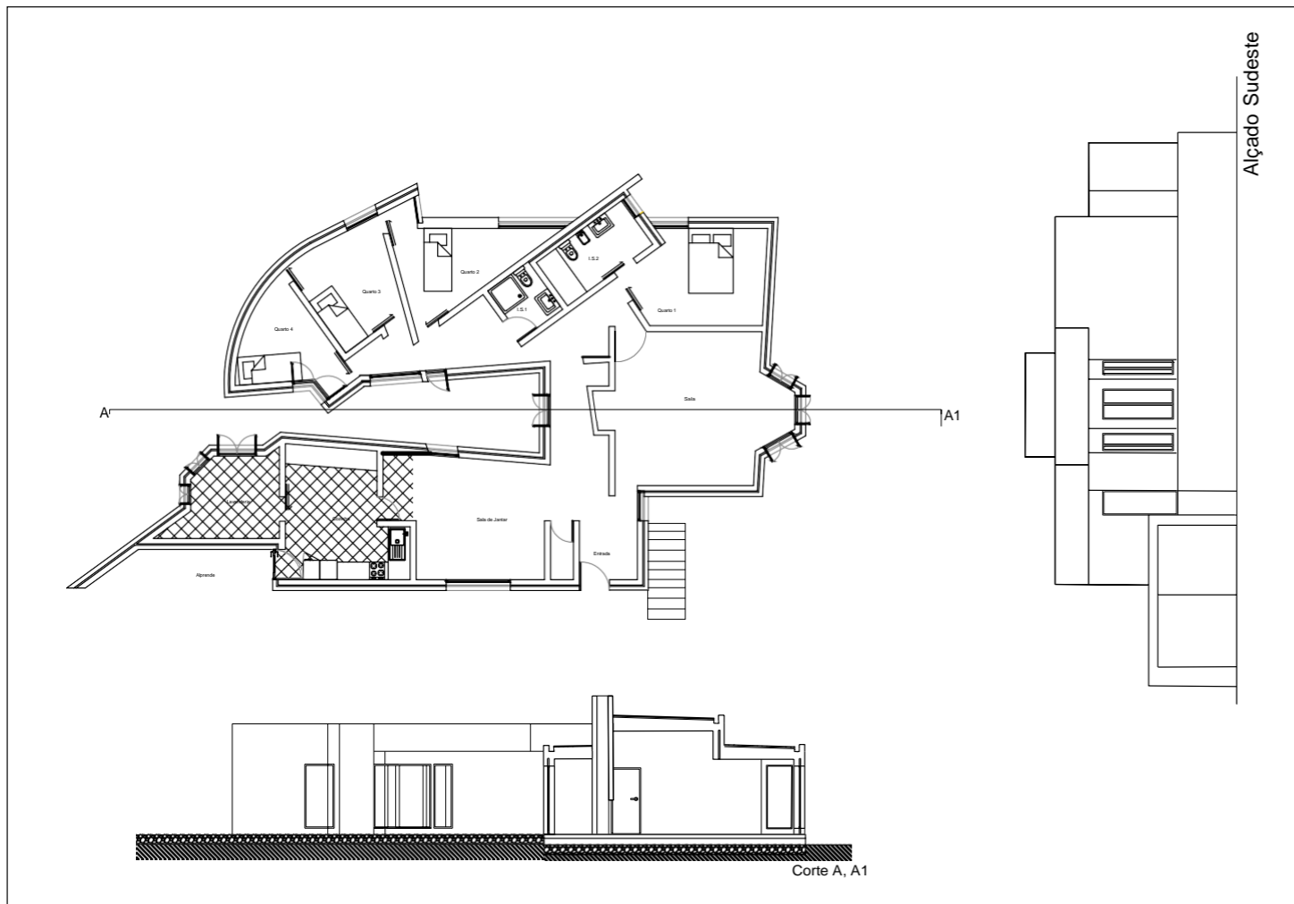
PLANTA, CORTE, E ALÇADO À ESCALA 1:100
