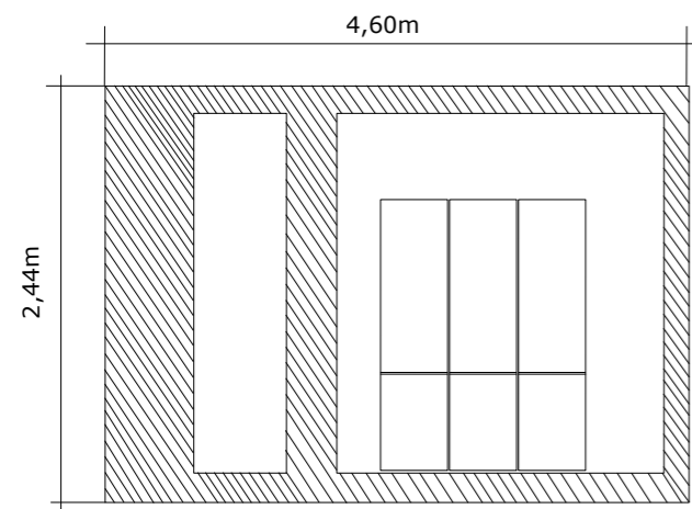
Corte Oeste
