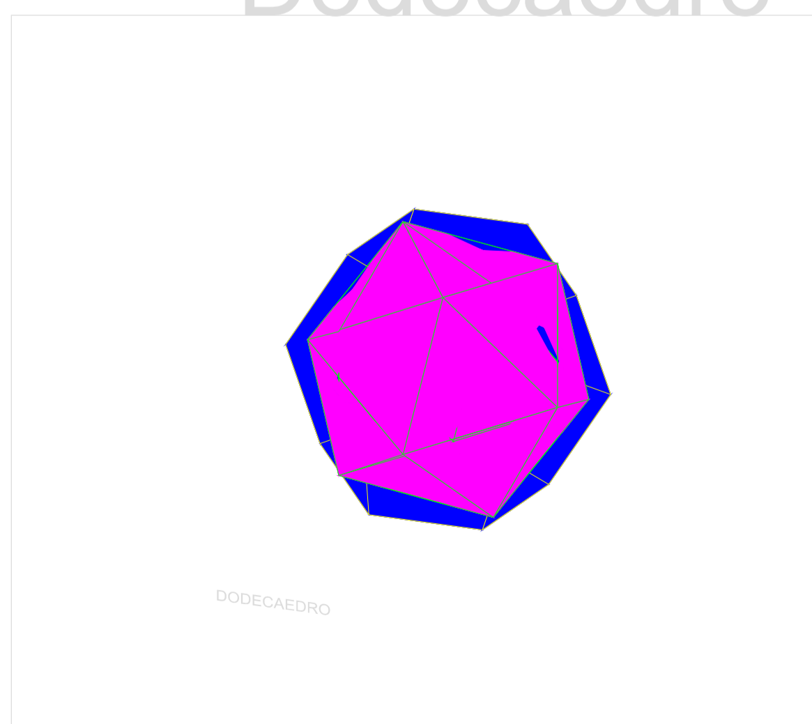
Dodecaedro
