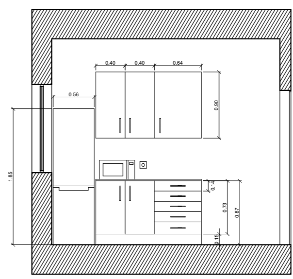
Corte B.2
