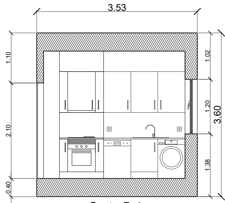
Corte B.1
