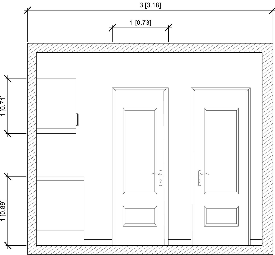
Corte CC`
