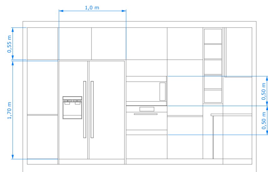
ALÇADO SUL
