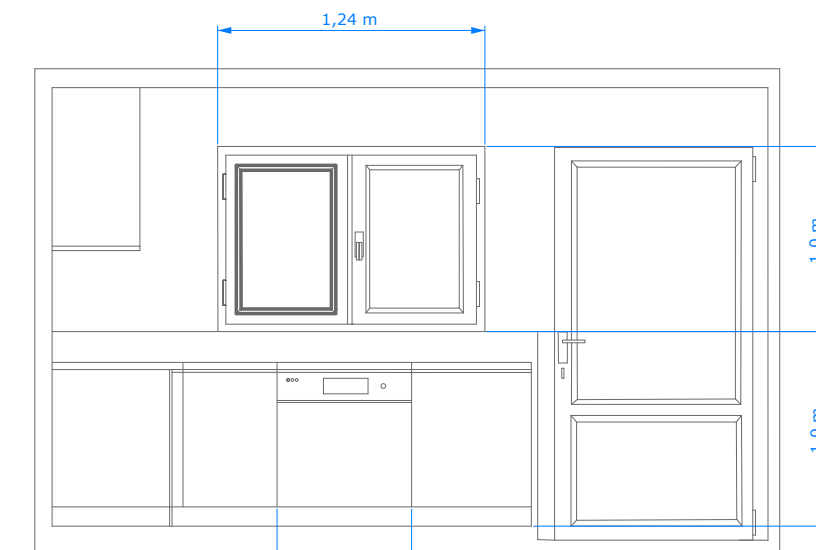
ALÇADO NORTE
