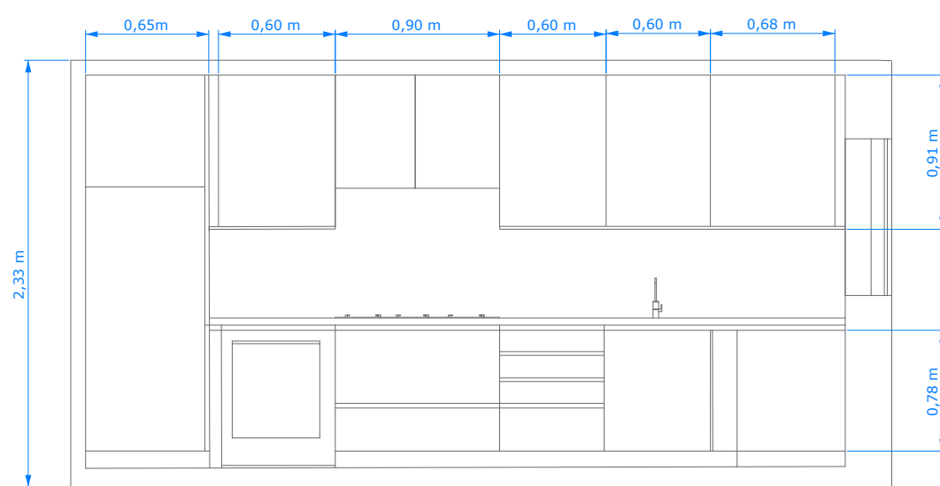
ALÇADO ESTE
