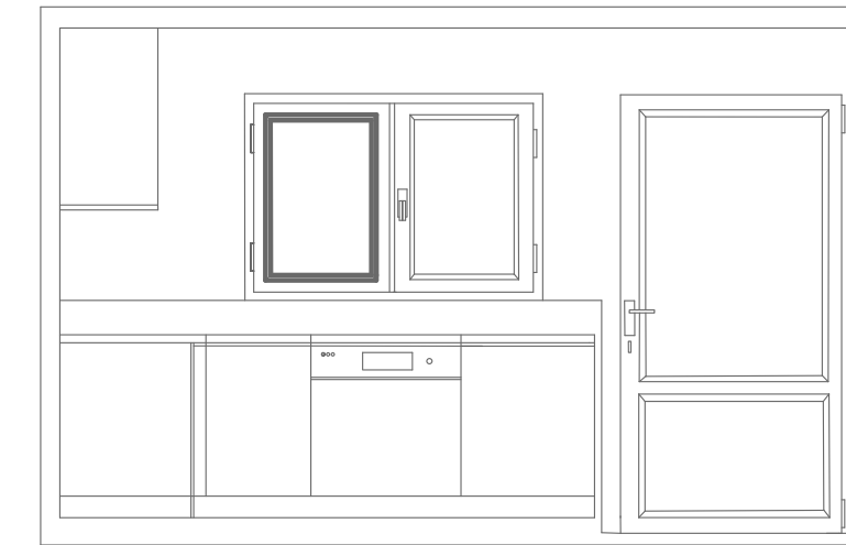
ALÇADO NORTE
