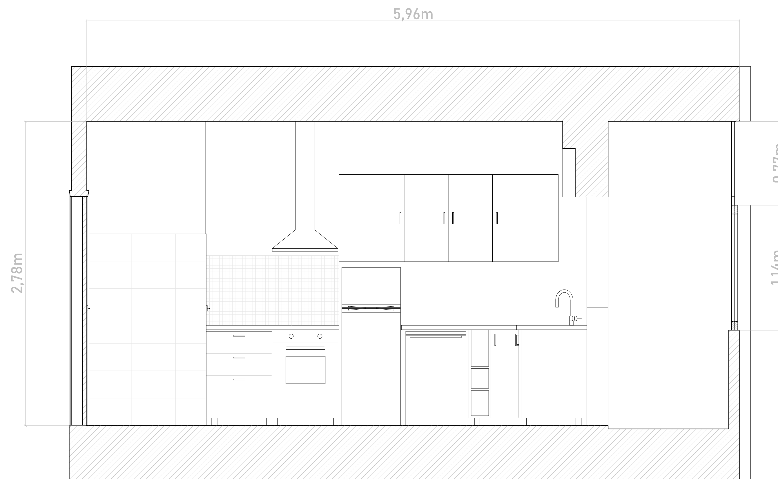
Corte AA'
