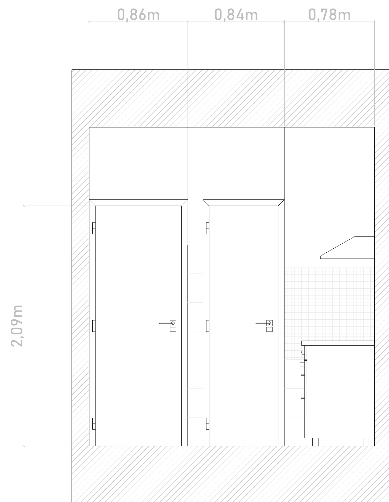
Corte BB'
