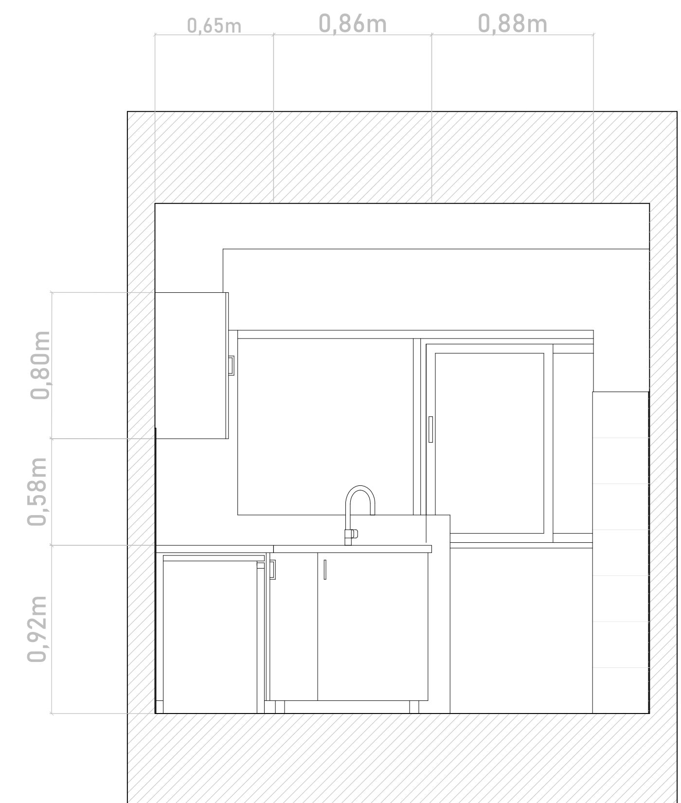
Corte CC'
