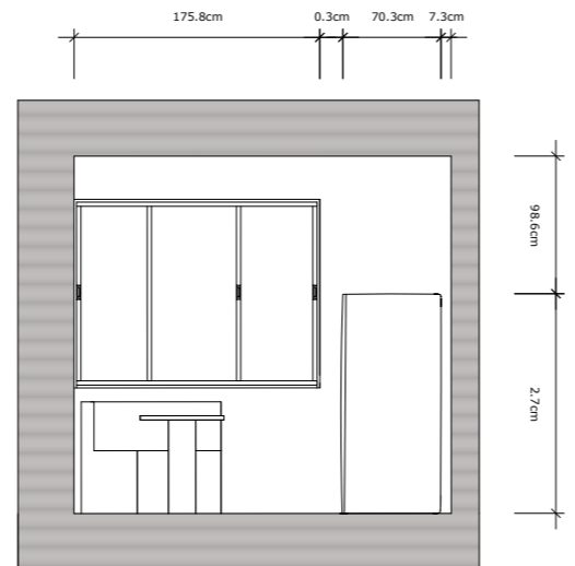
CORTE SUL
