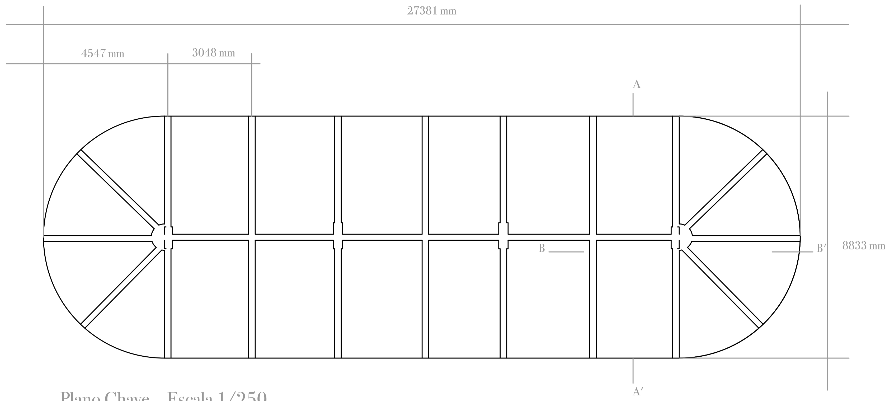
Plano Chave _ Escala 1/250
