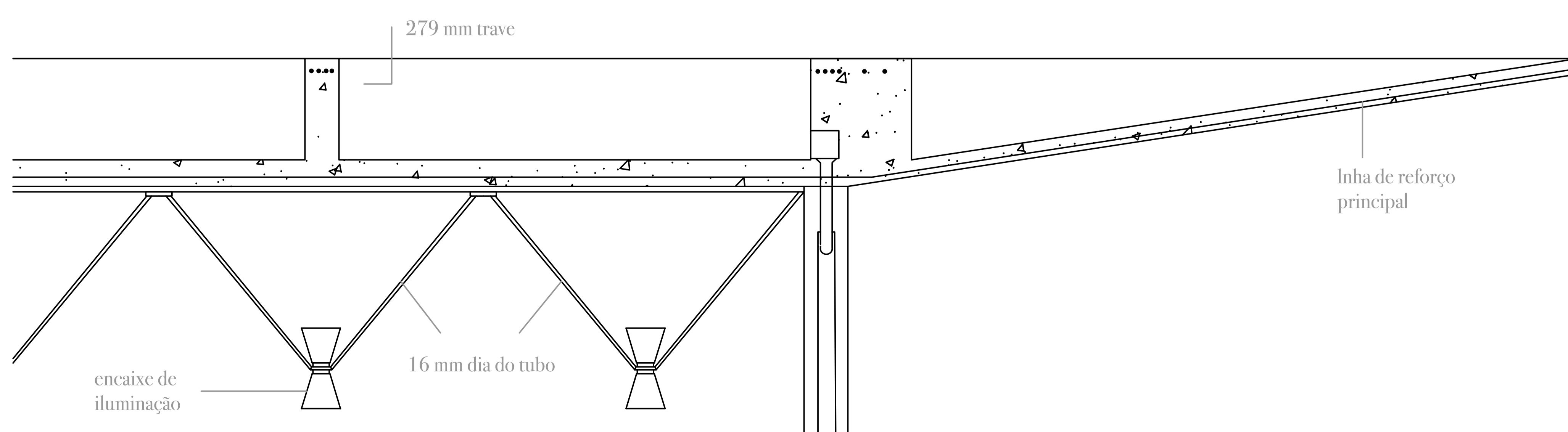
Secção BB' _ Escala 1/50
