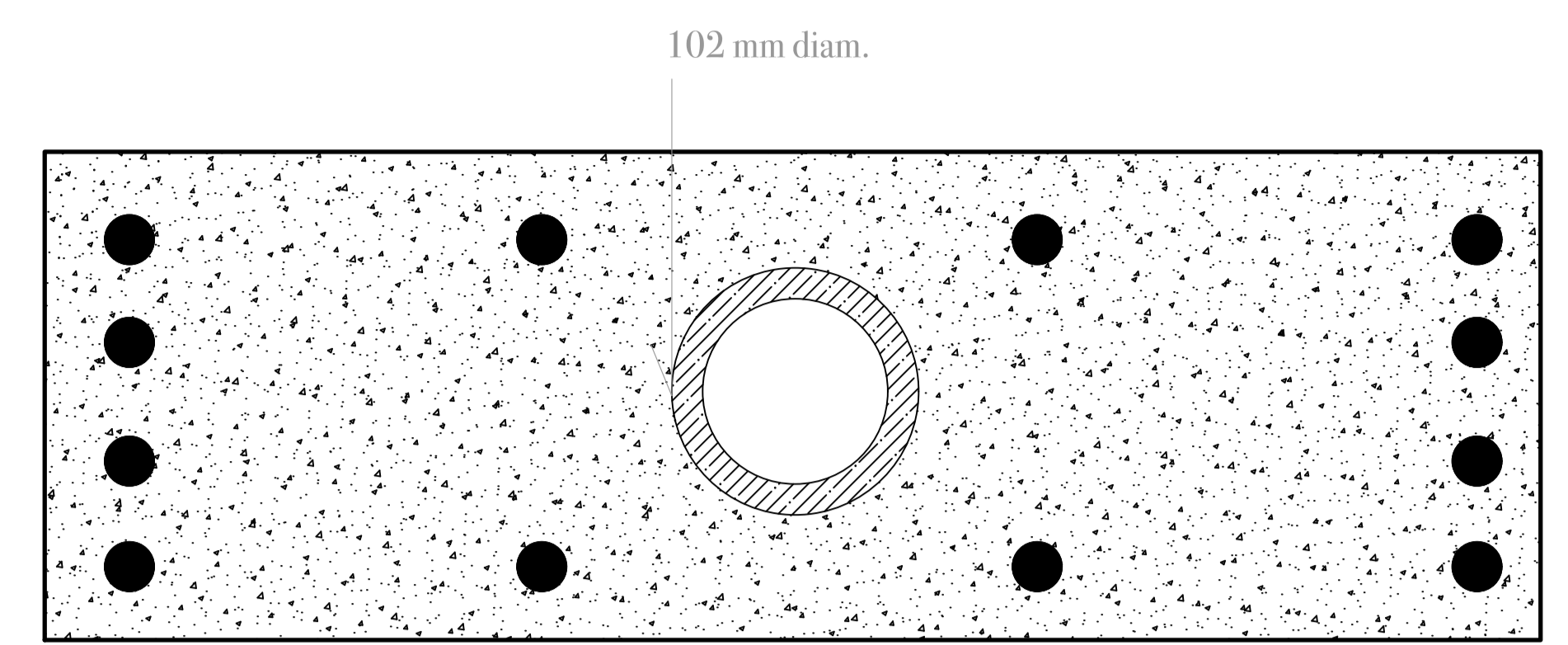
Plano de Coluna _ Escala 1/10
