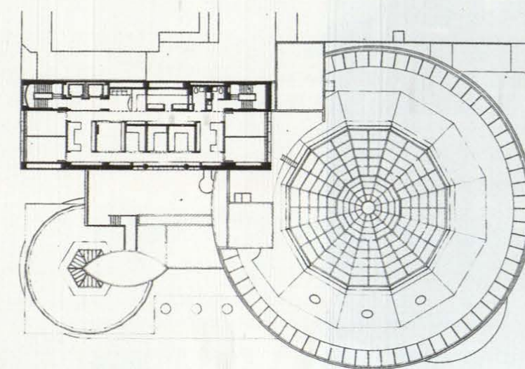
Planta novena 1 Administración
