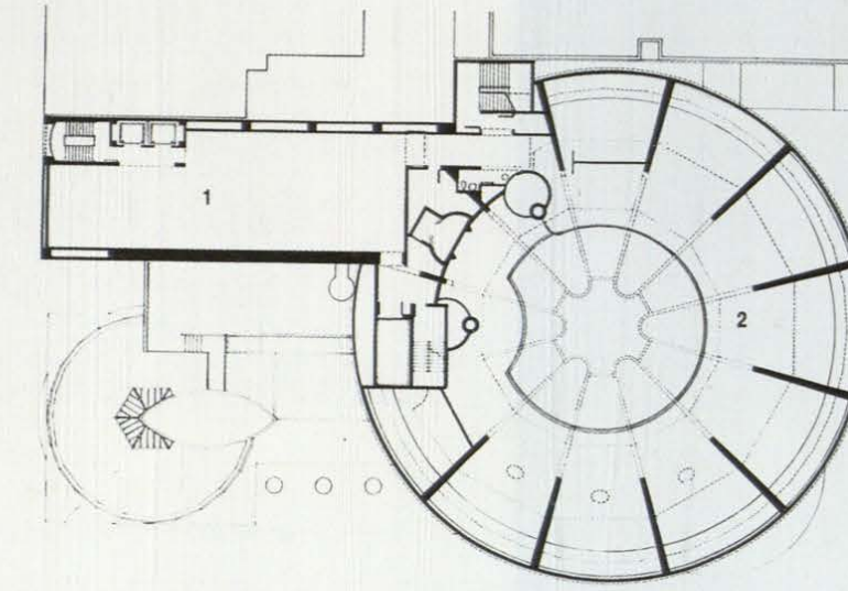
Planta séptima 1 Colección permanente 2 Exposiciones temporales
