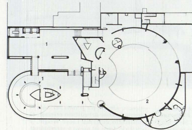
Planta segunda 1 Colección permanente 2 Exposiciones temporales
