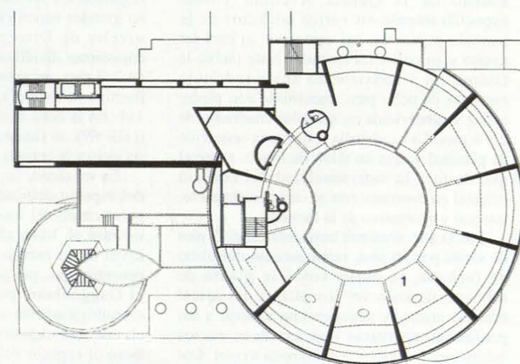
Planta sexta 1 Exposiciones temporales
