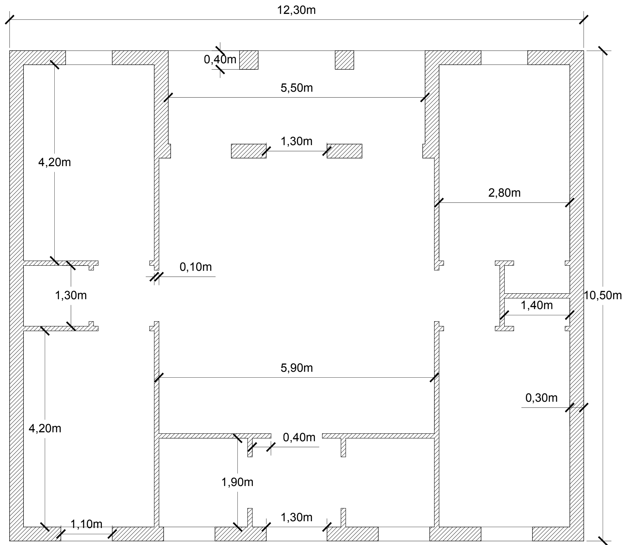
Planta do Rés-do-chão, escala 1:50
