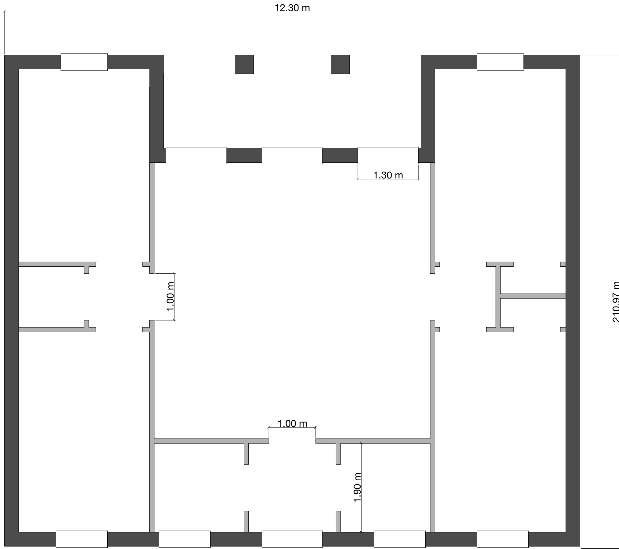
Planta R/C . Escala 1:50
