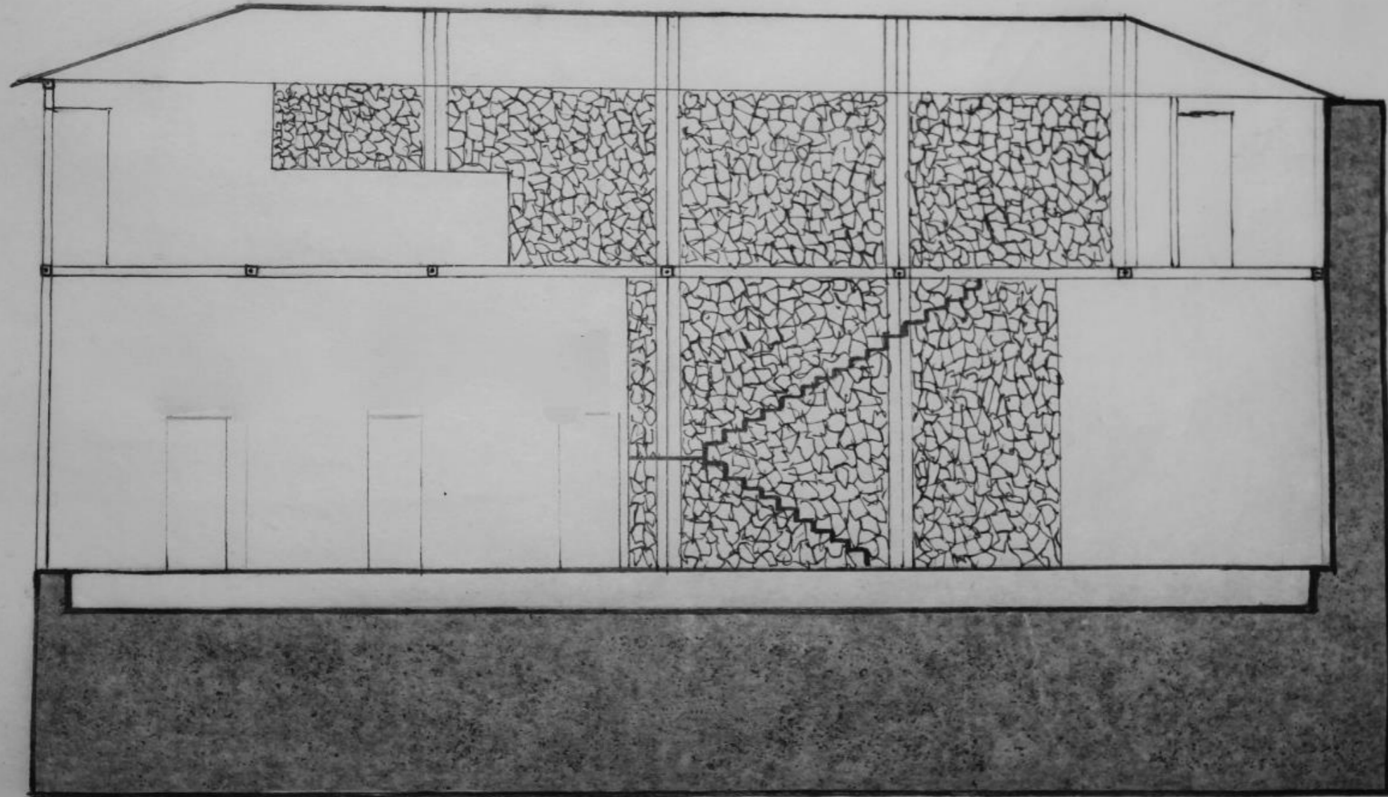
Corte B
