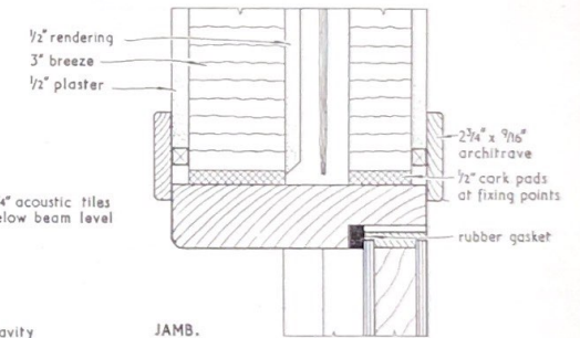
JAMB.
