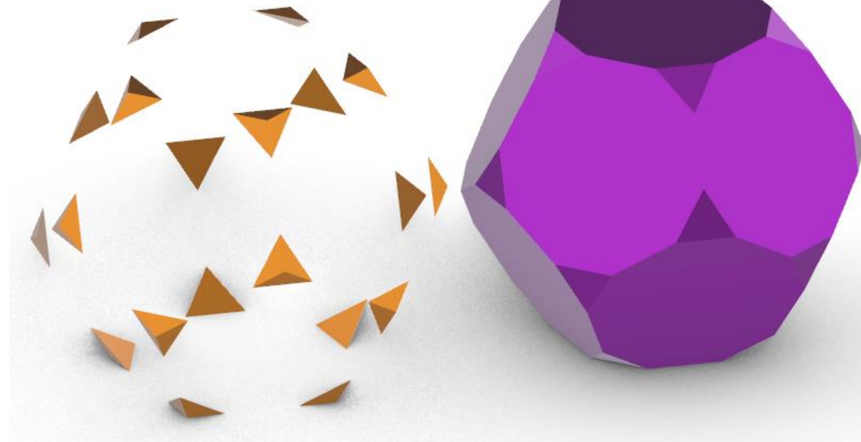
Exerc. 2.1 - Dodecaedro
