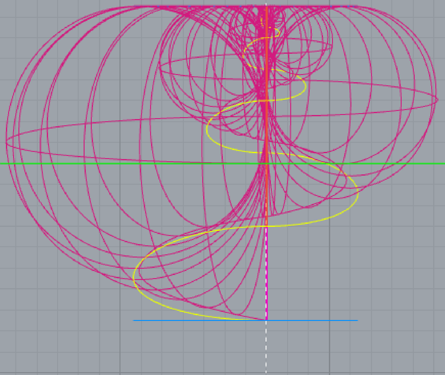
Ex:2.4 - Caracol
