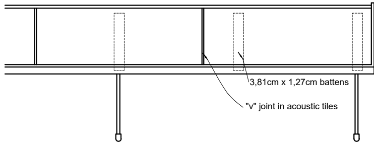
ELEVATION
