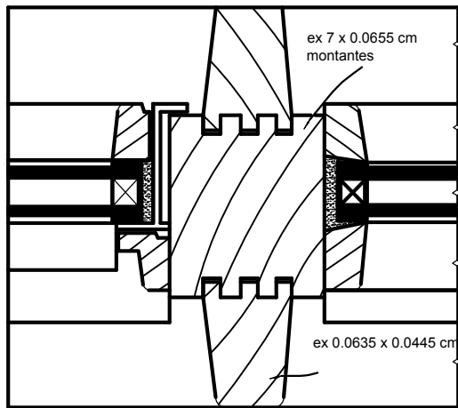
PLANO escala 1/2
