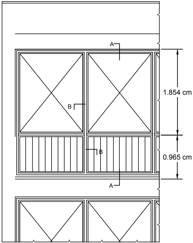
ELEVAÇÃO escala 1/50
